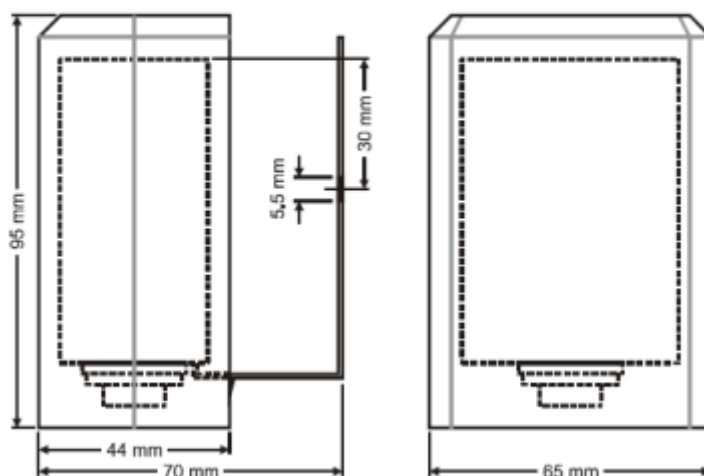
Fig. 1. Dimensions (mm)
